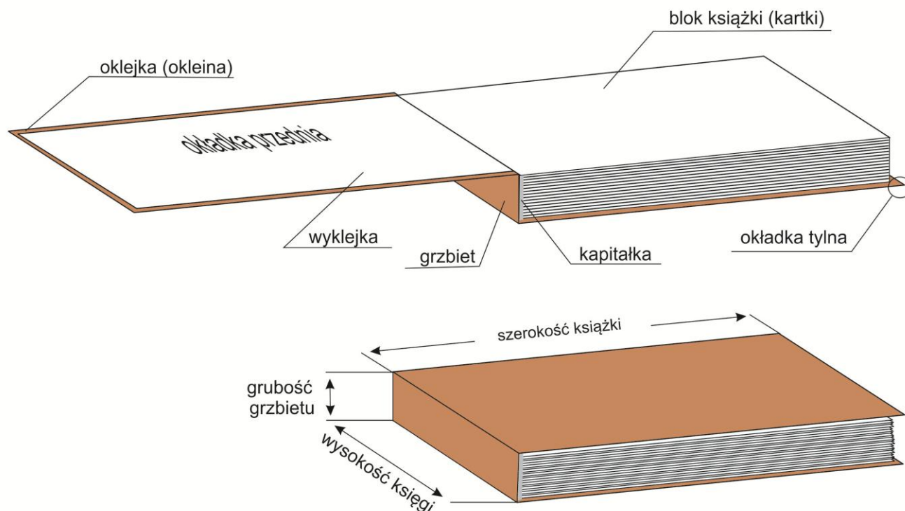
Rys. 1. Nazewnictwo w introligatorstwie
